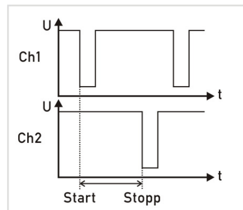
Prinzip zweikanalige Messung PNP
