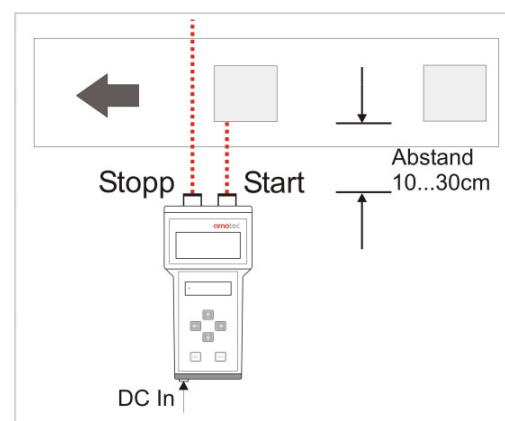
Anwendungsbeispiel einer Zweikanal Messung
