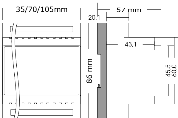
Masszeichnung
